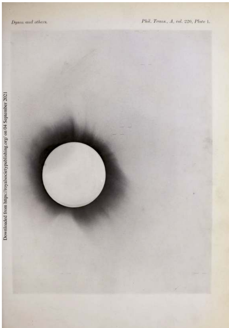
Abbildung 1: Halbtonreproduktion eines der in Sobral aufgenommenen Negative der Sonnenfinsternis vom 29. Mai 1919
