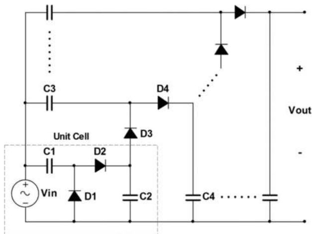
Figure 8. Karthaus-Fischer cascade voltage multiplier circuit.
