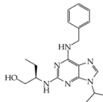
R-roscovitine (seliciclib) (CYC202)
