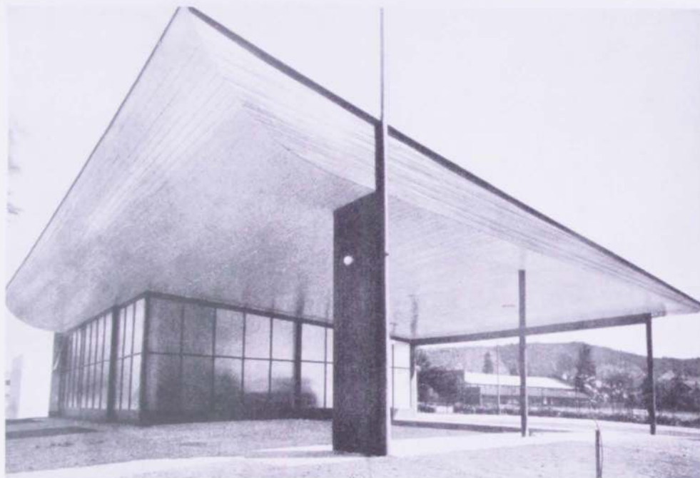
36. Jacques Groag, Tankstelle in Brunn/Brno, CZ, um 1937/38
